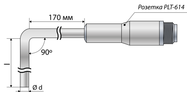
Рисунок Б.4 ПТСВ-3Г, ПТСВ-4Г
