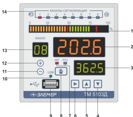
Передняя панель ТМ 5103Д
