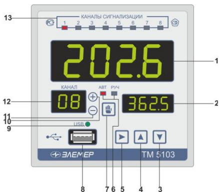
Передняя панель ТМ 5103
