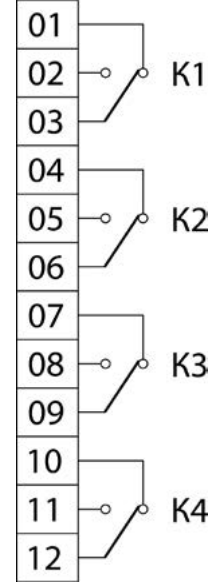
Модуль из 2-х токовых входов и 2-х токовых входов от расходомеров (код заказа «PT2»)
