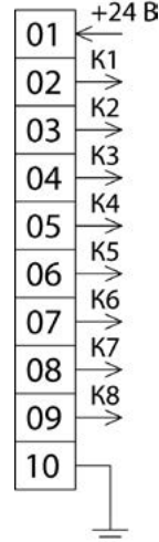
Интерфейсный модуль (код заказа «И2»)
