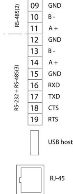
Интерфейсный модуль (код заказа «И2»)
