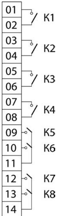
8-канальный модуль реле с нормально-разомкнутыми контактами (код заказа «P8»)
