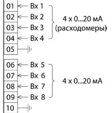
Модуль из 4-х токовых входов и 4-х токовых входов от расходомеров (код заказа «PT4»)
