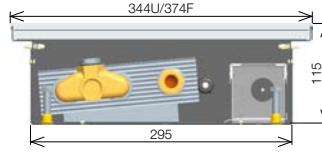
KORAFLEX FI 13/34 см. стр 62
