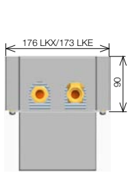
KORALINE LK ширина 18 см высота 9 см
