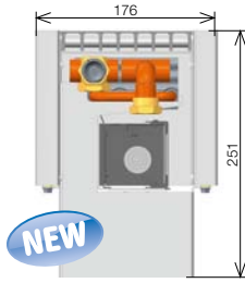
KORALINE LV 15/18 см. стр 74
