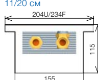
KORAFLEX FK 11/20 см
