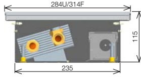
KORAFLEX FI 11/20 см. стр 61
