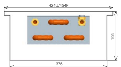
KORAFLEX FK 45/42 см
