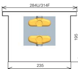
KORAFLEX FK 30/42 см
