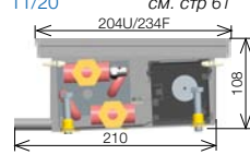
KORAFLEX FI 11/20 см. стр 61
