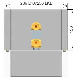
KORALINE LK ширина 24 см высота 15, 30, 45 и 60 см
