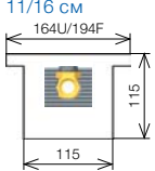
KORAFLEX FK 11/16 см
