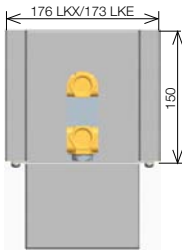
KORALINE LK ширина 18 см высота 15, 30, 45 и 60 см
