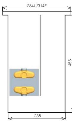
KORAFLEX FK 45/28 см
