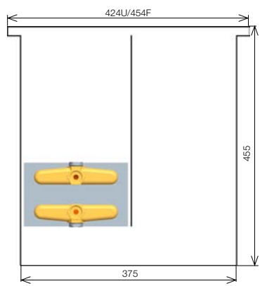
KORAFLEX FK 45/42 см
