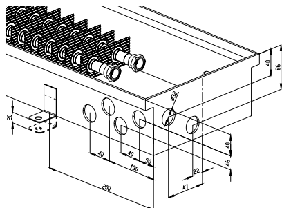
KORAFLEX FI 11/20 KORAFLEX FV 11/20
