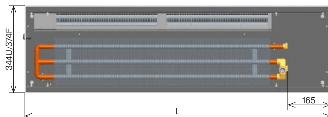
Размеры указаны в мм с U и F-образными рамками.
