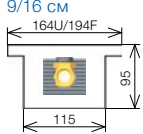
KORAFLEX FK 9/16 см
