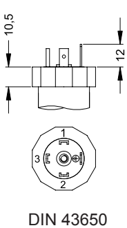
DIN 43650
