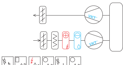
Схема 3.2 VAC-EO-ShD1D3D35D125Te
