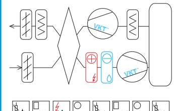
Схема 3.6 VAC-W-ShD1D3D35D35D125Te
