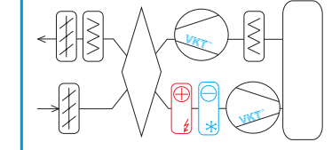
Схема 6.6 VAC-EF-ShD1D1D3D3D35D35D125TeKt
