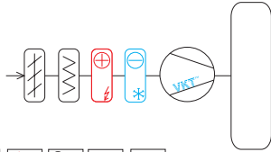
Схема 6.1 VAC-EF-ShD1D3D35D125TeKt
