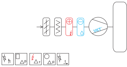
Схема 3.1 VAC-EO-ShD1D3D35D125Te
