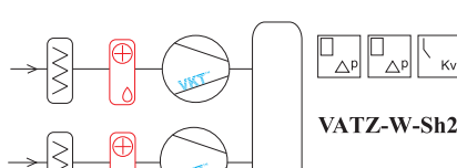
VATZ-Sh2D1D1Kv
