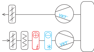
Схема 6.2 VAC-EF-ShD1D3D3D35D125TeKt
