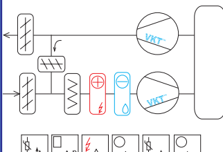
Схема 3.3 VAC-W-ShD1D3D35D125Te
