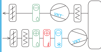
Схема 6.5 VAC-EF-ShD1D1D3D3D35D35D125TeKt
