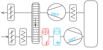
Схема 6.4 VAC-EF-ShD1D1D3D3D35D35D125TeKt
