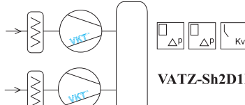
Схема 7.2 Воздушно-тепловая завеса с двумя вентиляторами
