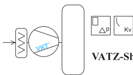
Схема 7.1 Воздушно-тепловая завеса с одним вентилятором
