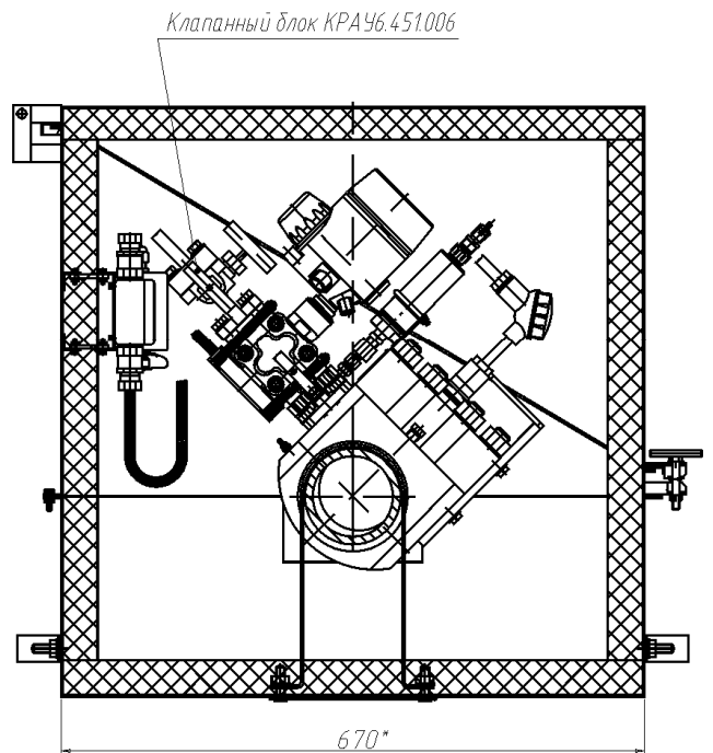
Вариант A-A (модель 250M с клапанным блоком)
