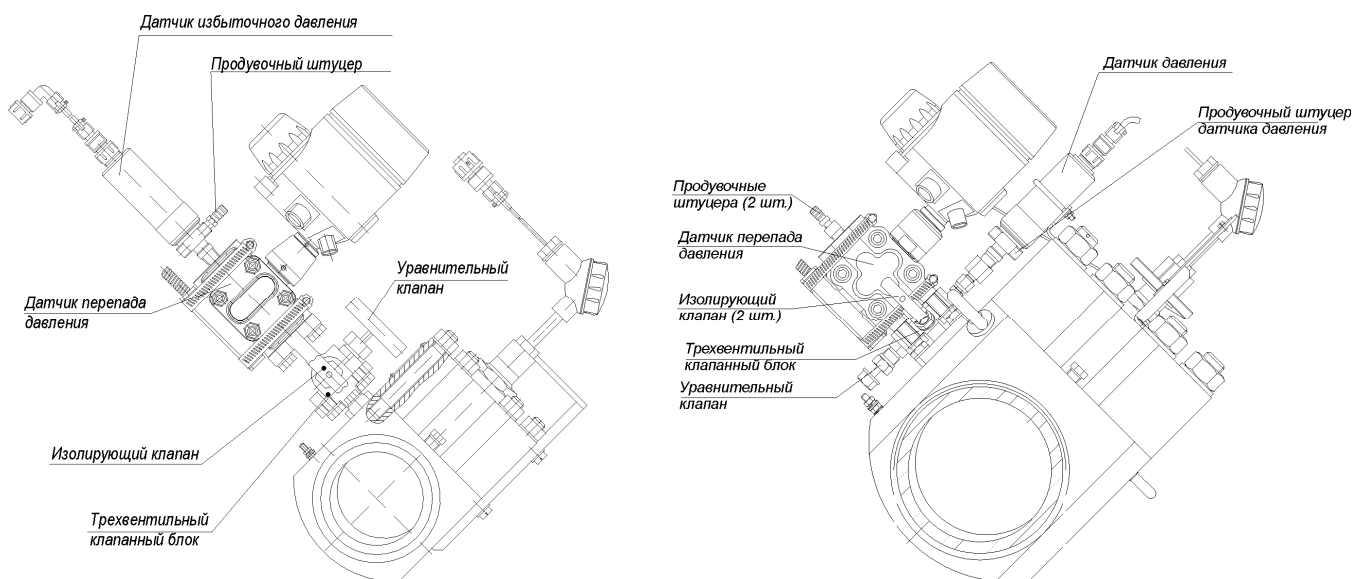
а) Модели 160, 160Ф, 250 и 250Ф
