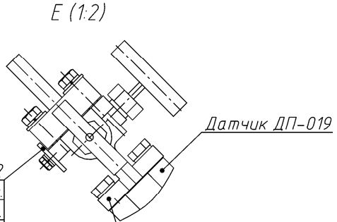
а) для расходомеров КРАУ2.833.006
