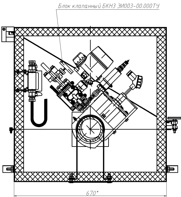
Вариант A-A (модель 160M с клапанным блоком)
