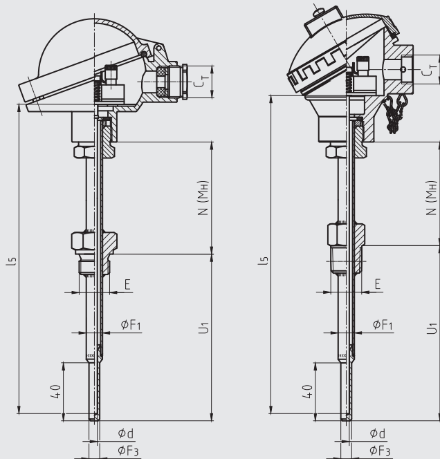
цилиндрическая резьба
