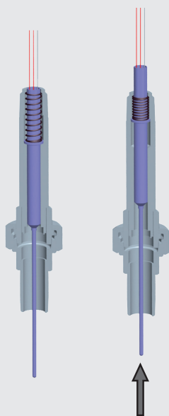
Иллюстрация хода пружины при монтаже (на примере модели TC12-M)
