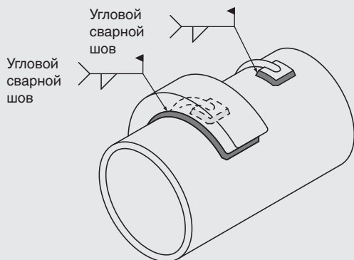
Рисунок 1: Схема сварки
