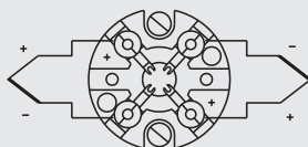
Сдвоенная термопара
