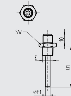
Rundstecker M12 x 1
