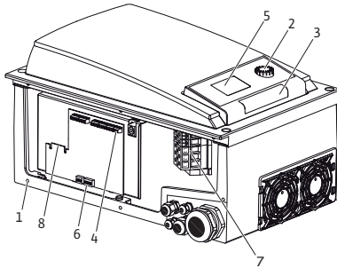
Рис. 9: Электронный модуль
