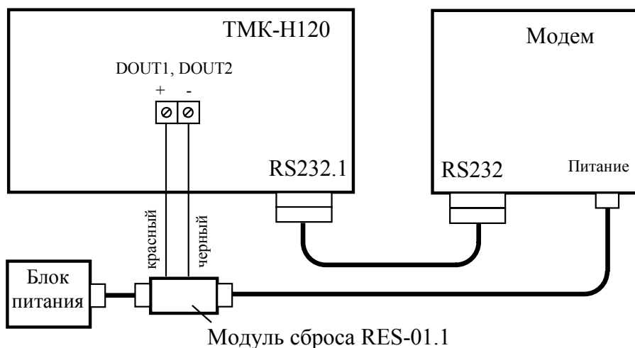
Подключение вычислителя к модему и блоку питания с использованием модуля сброса
