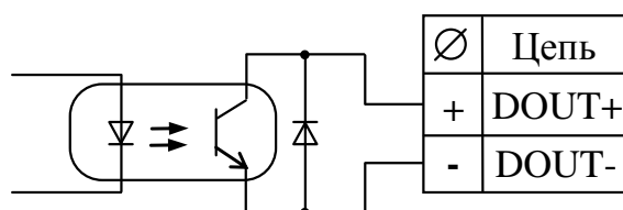
Организация дискретных выходов
