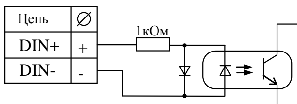
Организация дискретных входов
