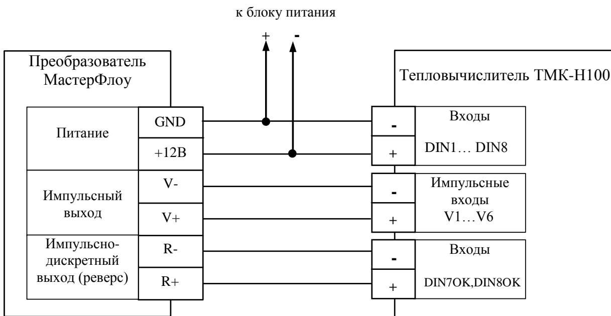
Пример подключения преобразователя МастерФлоу с импульсным выходом к ТМК-Н100 с обеспечением контроля напряжения питания и изменения направления потока
