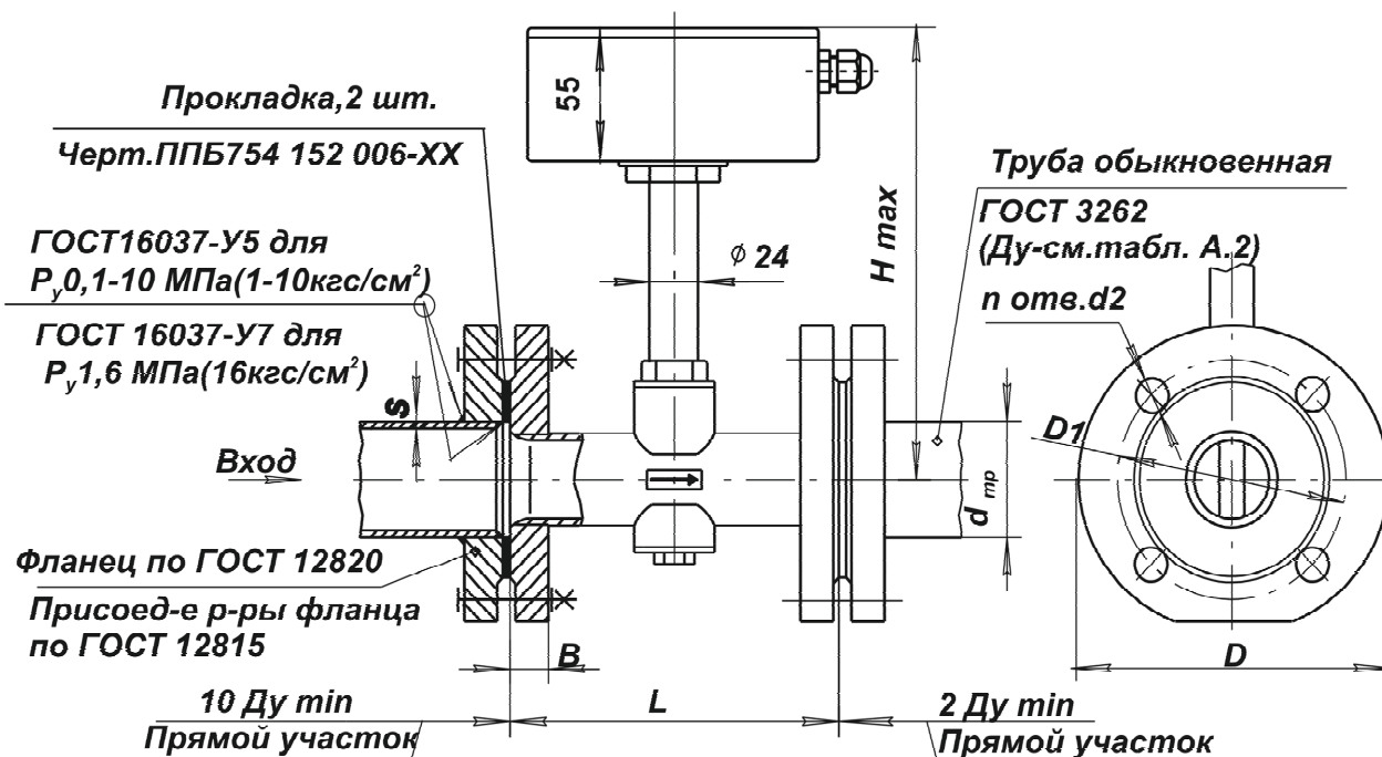
Рисунок А.1 – Габаритные и присоединительные размеры преобразователей ВПС3-ЧИ2.34
