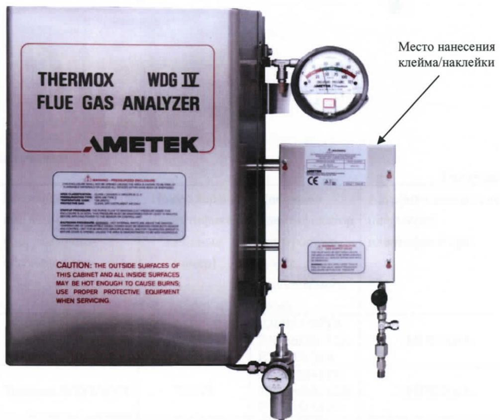
Рисунок 1 - Газоанализаторы серии WDG-IV
