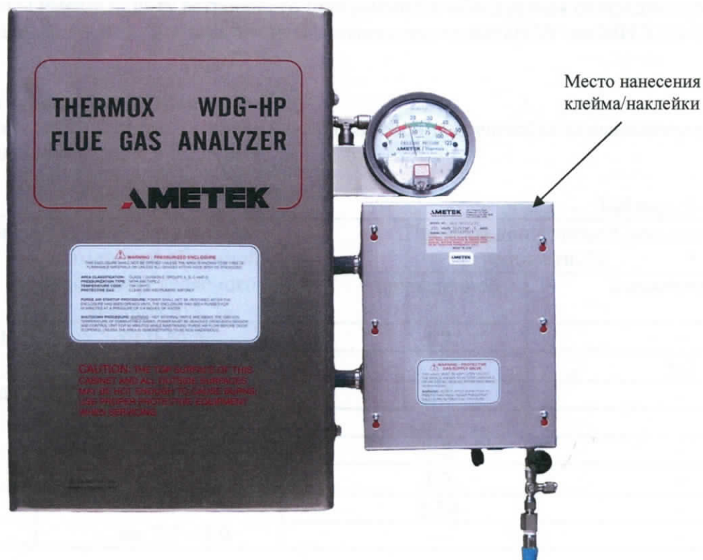
Рисунок 2 - Газоанализаторы серии WDG-HPII
