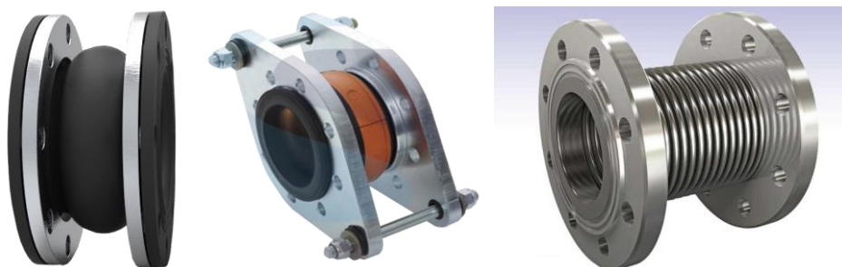
Рис. 15 Трубные компенсаторы
