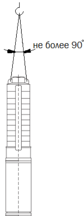
Рисунок 4 Схема строповки агрегата электронасосного
