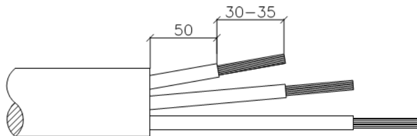
Рисунок 7. Оголение электрокабеля
