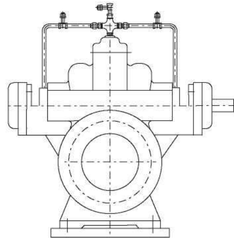
05 Промывочный водовод торцевого уплотнения с выпускным клапаном
