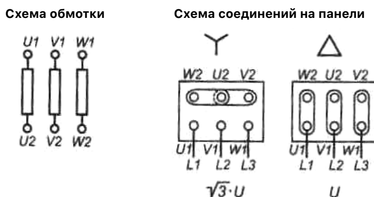
Рис. 2. Подключение электродвигателя
