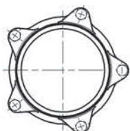
KRS-63 ホースカップリング図 (5点留め)
